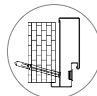
montážní otvor na kotvu na falci zárubně
