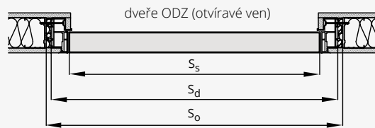
DVEŘE OTVÍRÁVÉ VEN ODZ
